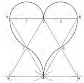
Trazado de la figura cordiforme
