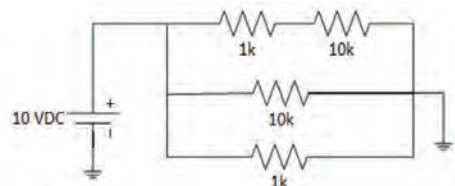
Figura 1: Esquema eléctrico del circuito ejemplo para trabajar la Ley de Kirchhoff
