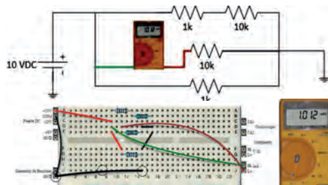
Figura 2: Ejemplo de medida de corriente en la rama intermedia del circuito.
