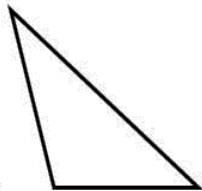
Obtusángulo Un ángulo obtuso
