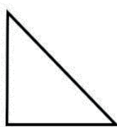
Rectángulo Un ángulo de 90^\circ
