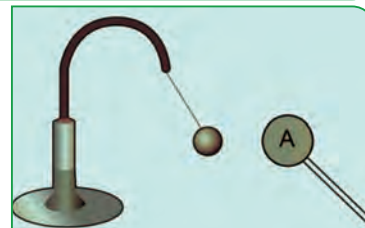
Figura b. Se aproxima uno al otro y sucede la inducción
