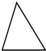
Acutángulo Los 3 ángulos son agudos
