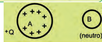
Figura a. Cuerpos antes del contacto.
