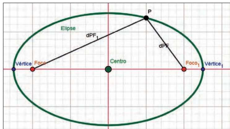
Figura 1: Elipse
