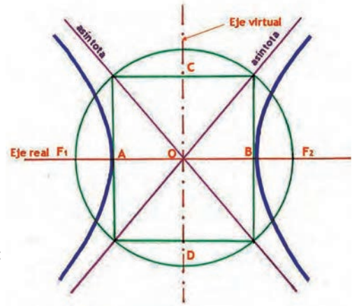
Figura 1: Hipérbola
