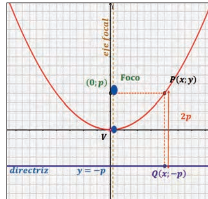
Figura 1: Parábola
